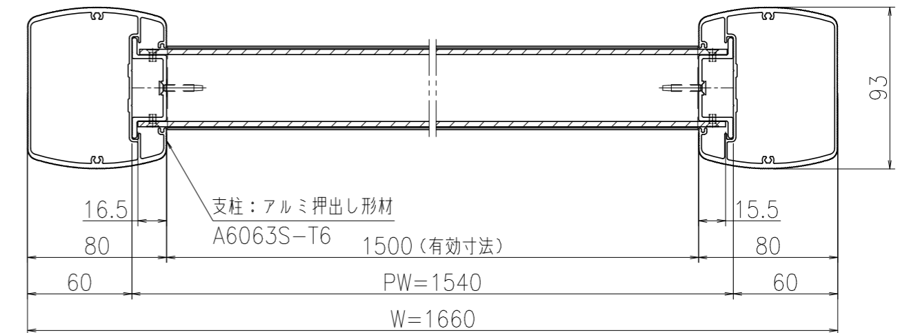
A-A'断面図 (S=1:3)
