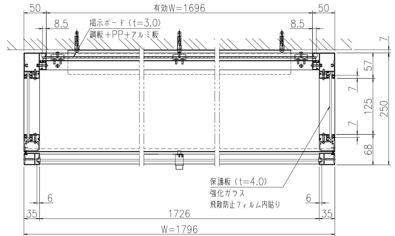
A-A'断面図（S=1：5）
