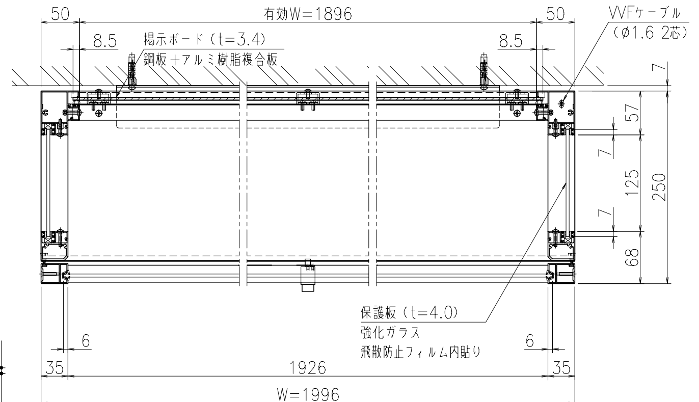
A-A'断面図（S=1：5）
