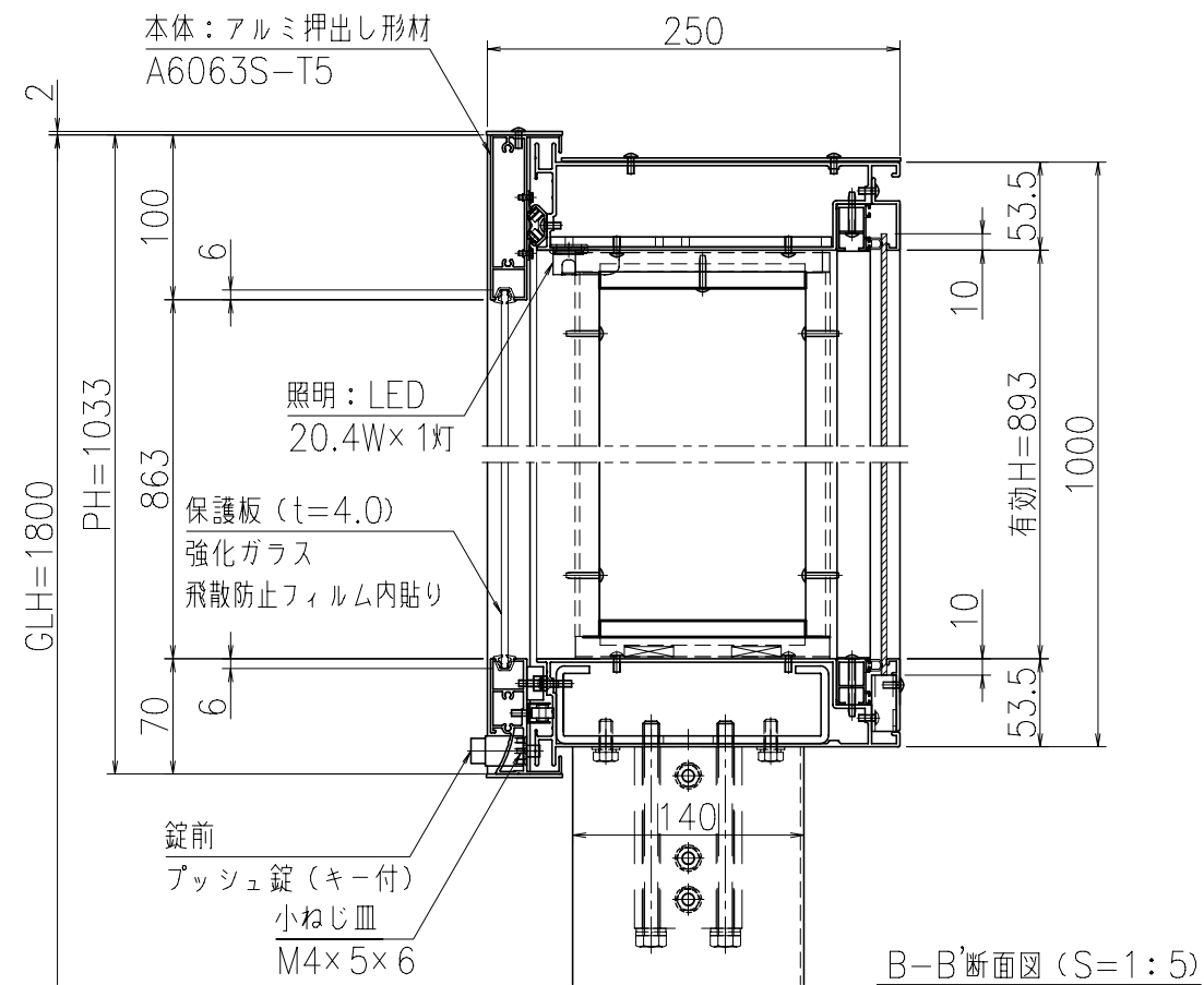
A-A'断面図（S=1：5）
