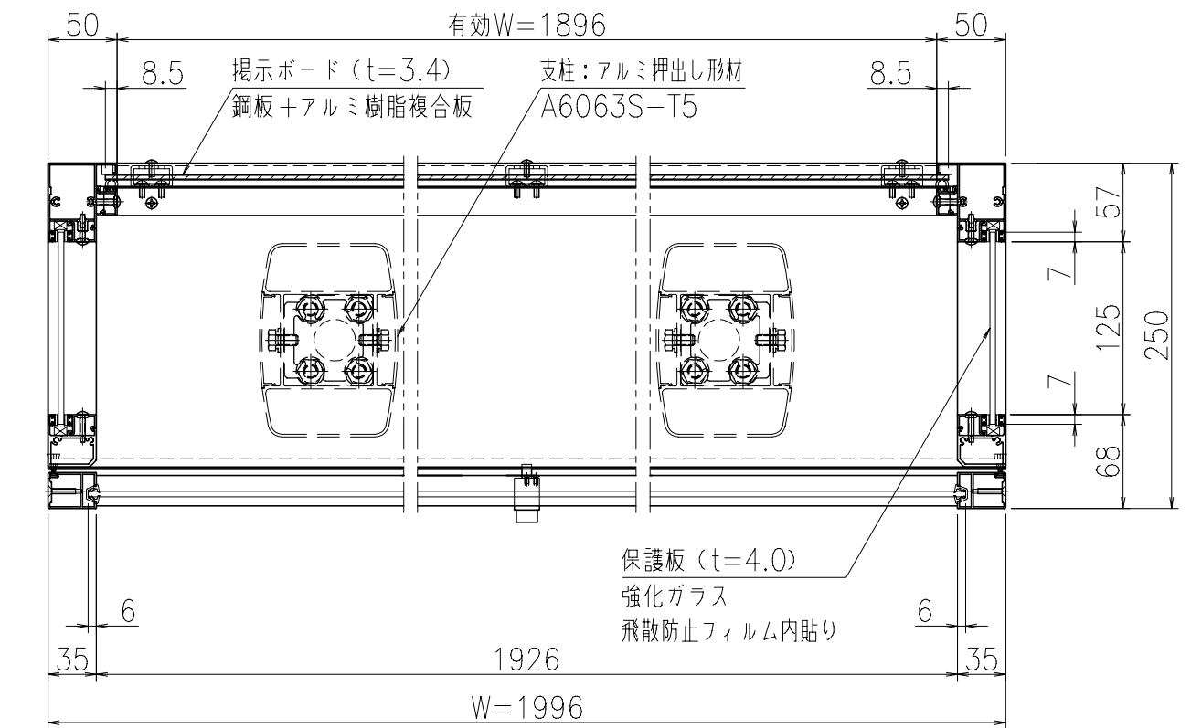
A-A'断面図（S=1：5）
