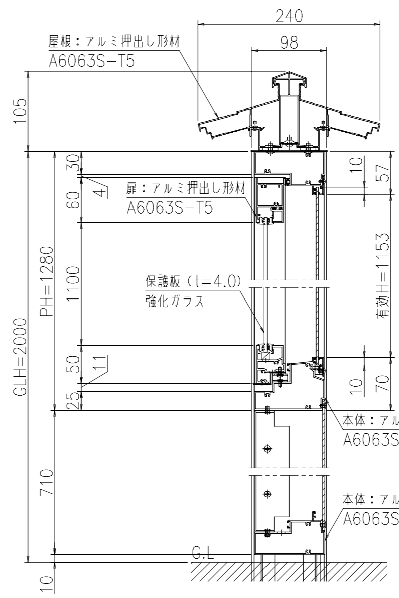
A-A'断面図 (S=1:5)
