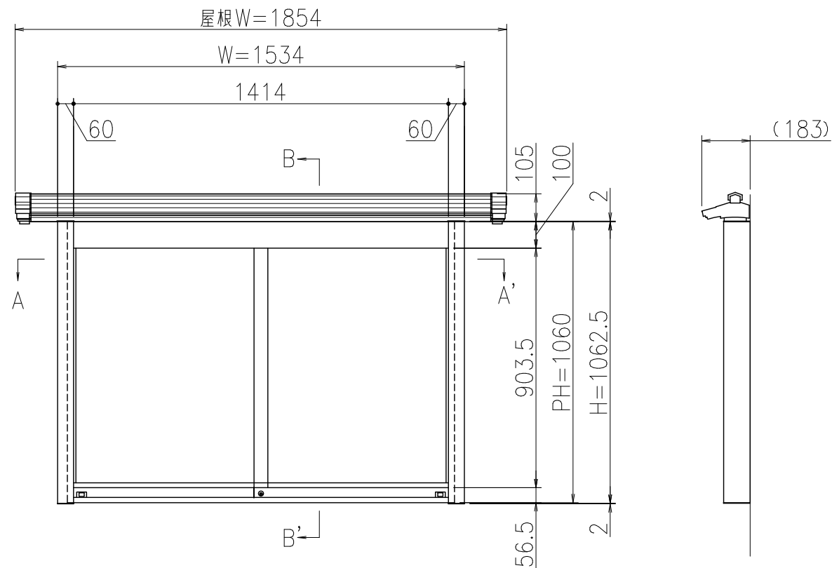
壁面取り付け穴寸法
