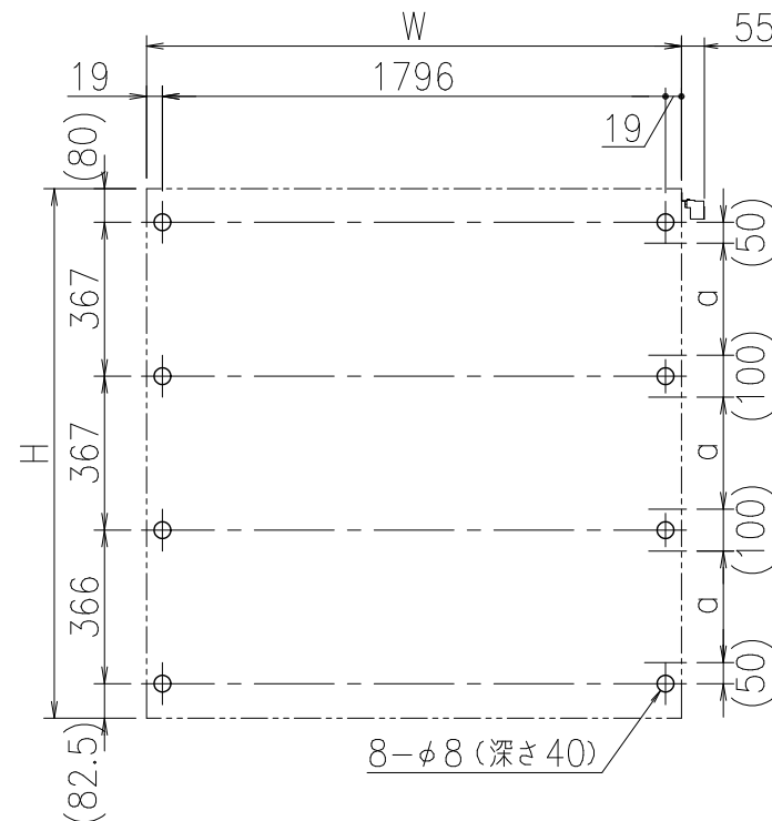
壁面取り付け穴寸法
