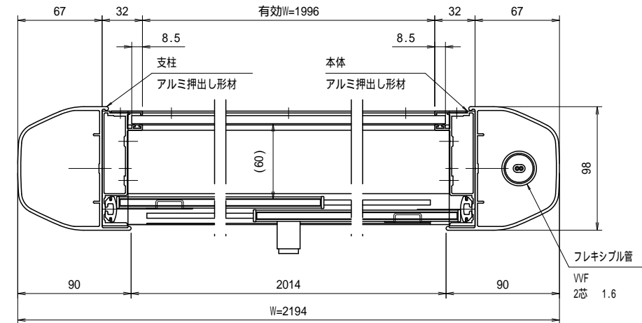
A-A' 断面図 (S=1:3)
