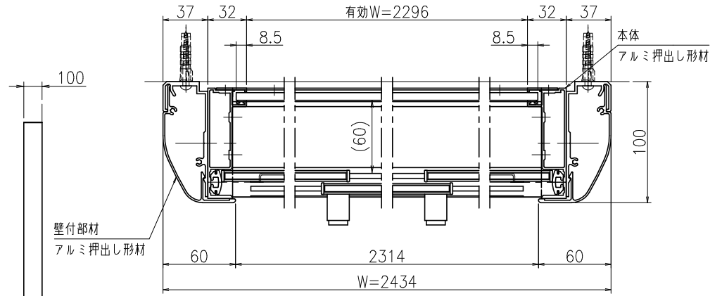
A-A断面図 (S=1:3)
