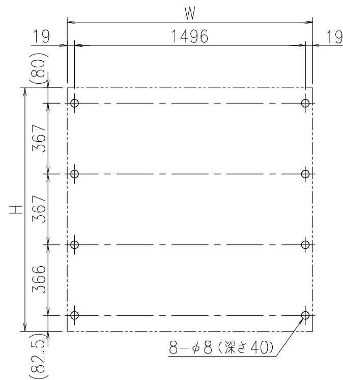
壁面取り付け穴寸法
