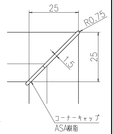
C部納まり図 (S=1:1)
