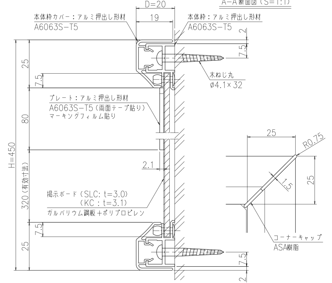
B-B'断面図 (S=1:1)
