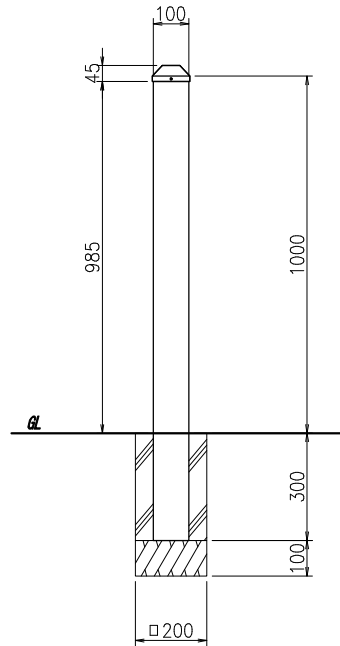
【正面図】
