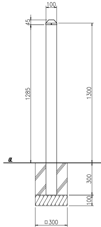
【正面図】
