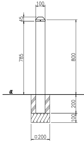
【正面図】
