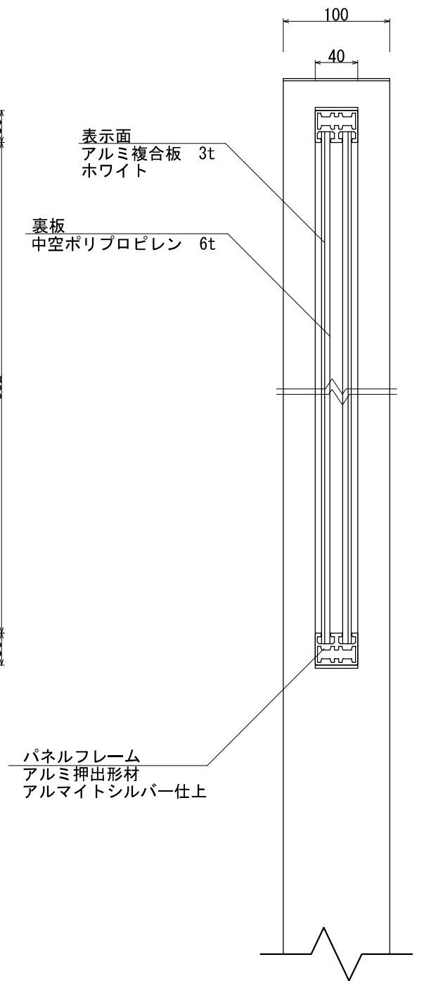
【側断面図】
